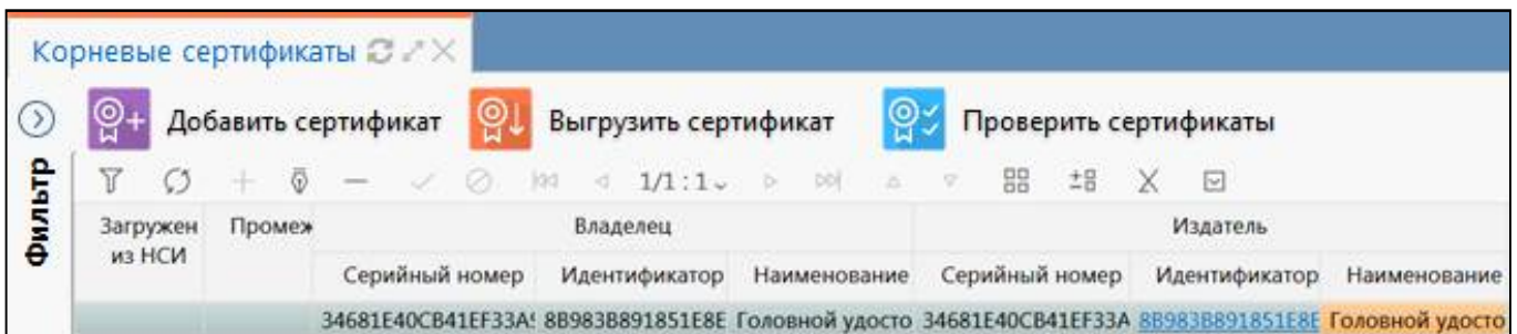
Рисунок 45 – Добавленный сертификат
