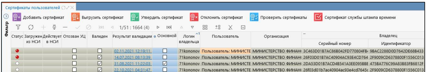
Рисунок 51 – Проверка сертификатов
