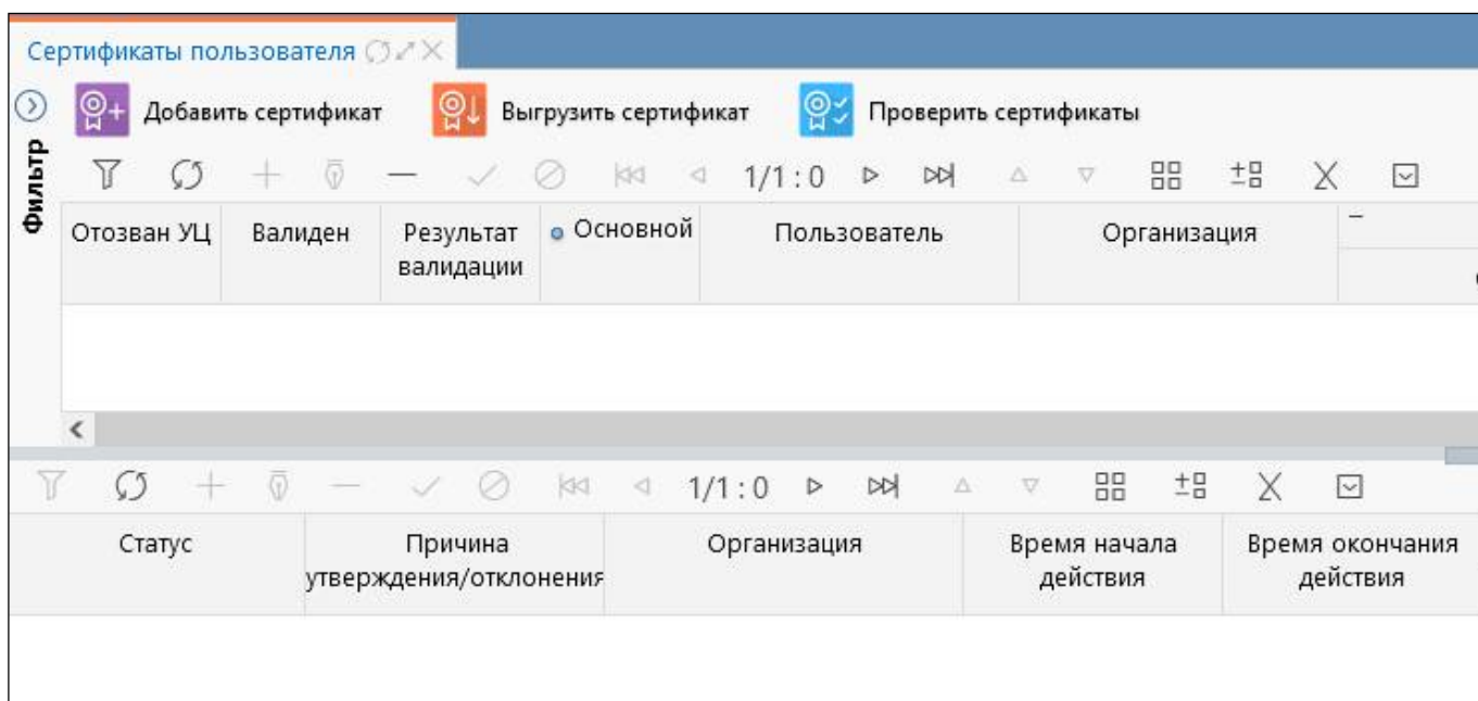
Рисунок 55 – Интерфейс «Сертификаты»
