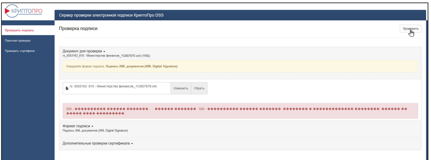
Рисунок 62 – Интерфейс «КриптоПро»
